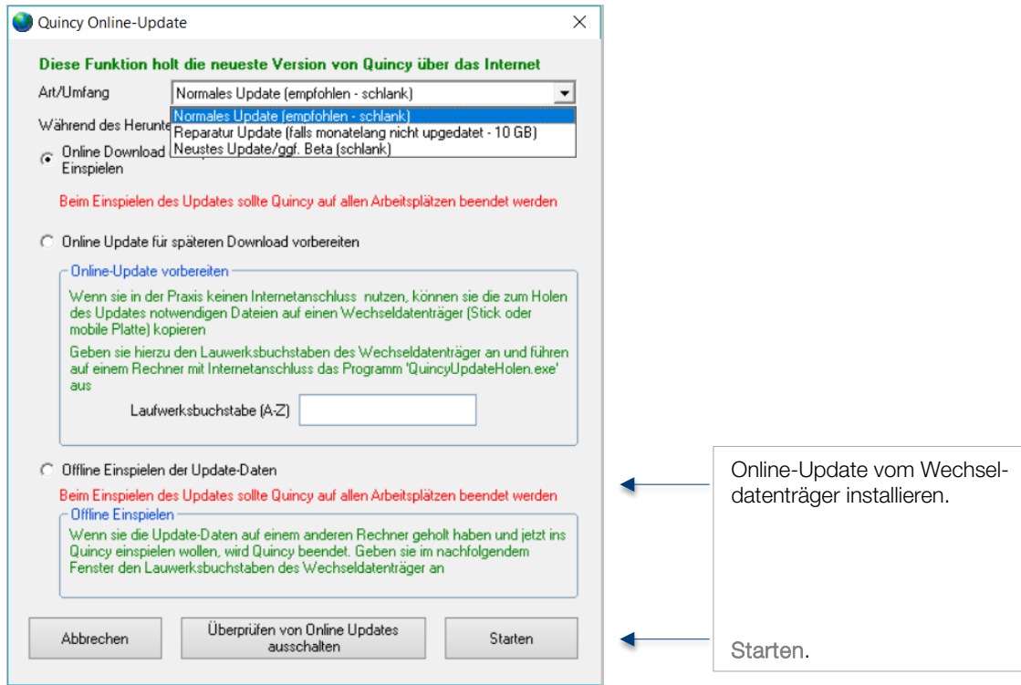
Abb. 10 Online-Update Einstellungen
