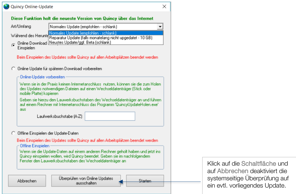
Abb. 12 Online-Update Einstellungen
