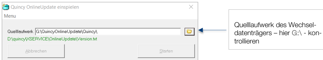
Abb. 11 Quelllaufwerk
