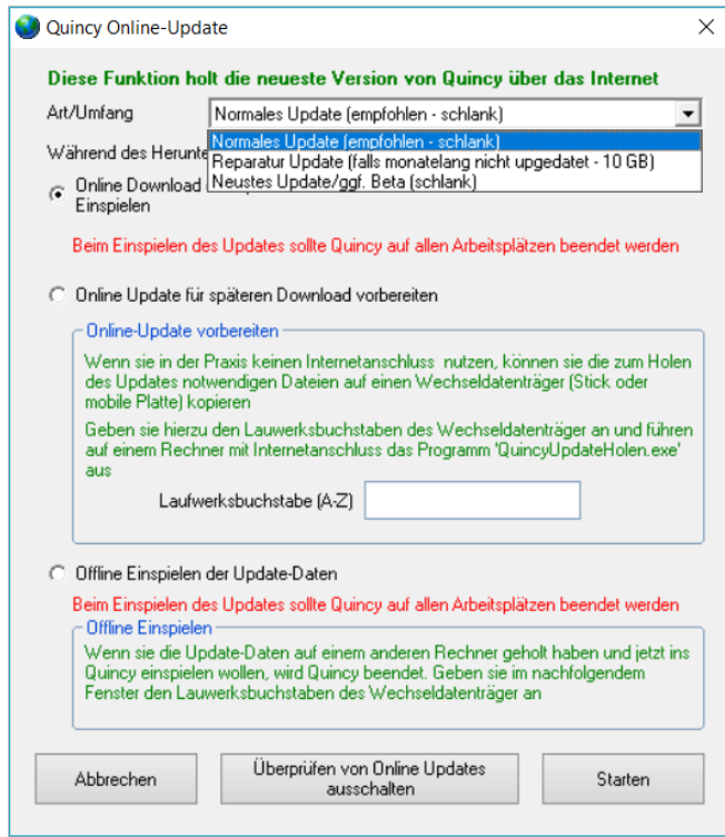
Abb. 9 Online-Update Einstellungen
