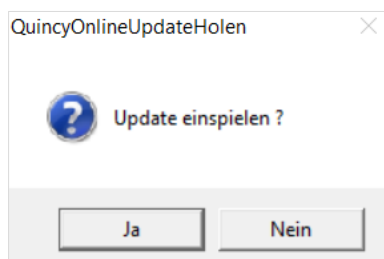
Abb. 7 Abfrage
