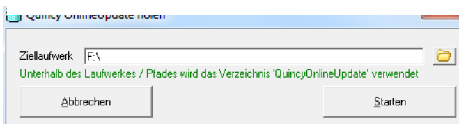
Abb. 4 Ziellaufwerk angeben
